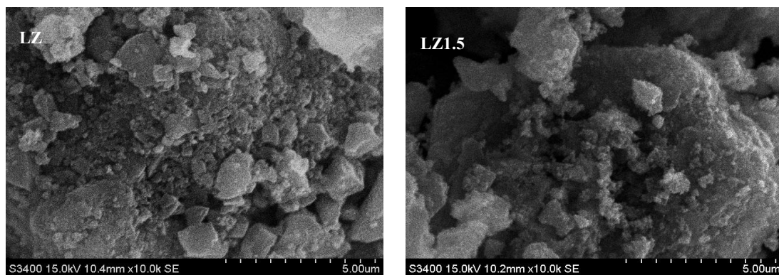
图 6 生物质炭的扫描电镜图( \times 10\,000 倍)
